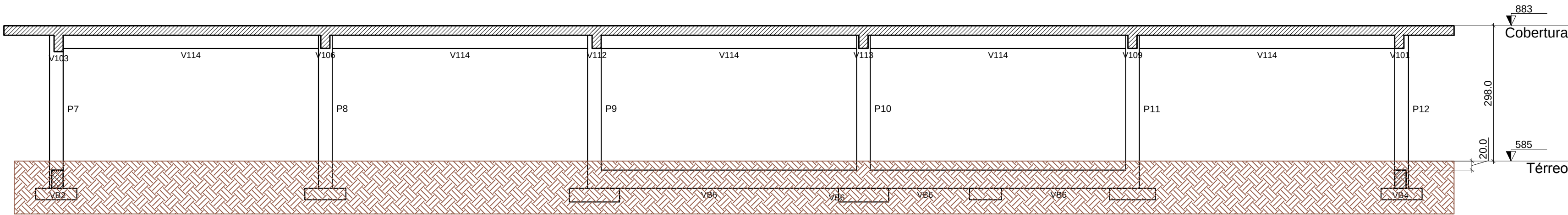
CORTE A-A ESC.1:75
